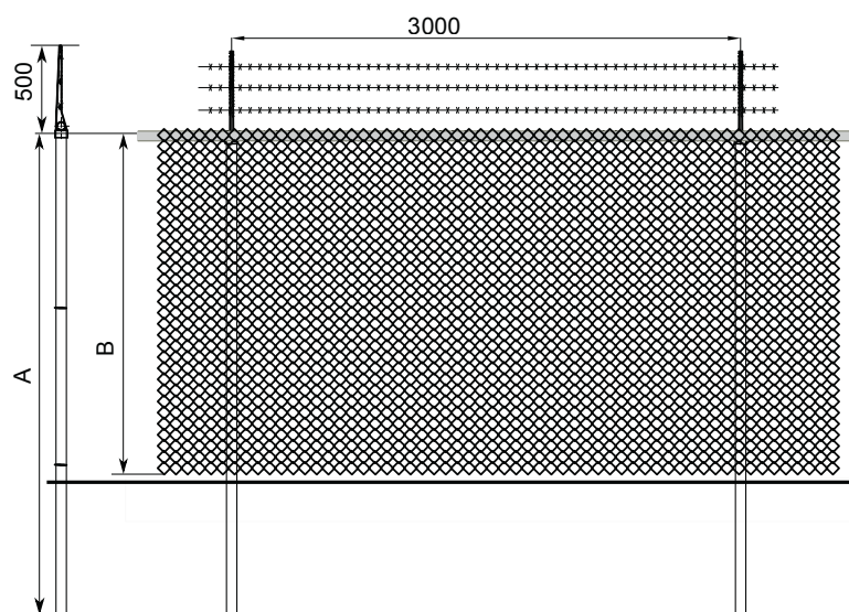
Rechte puntdraadhouder
